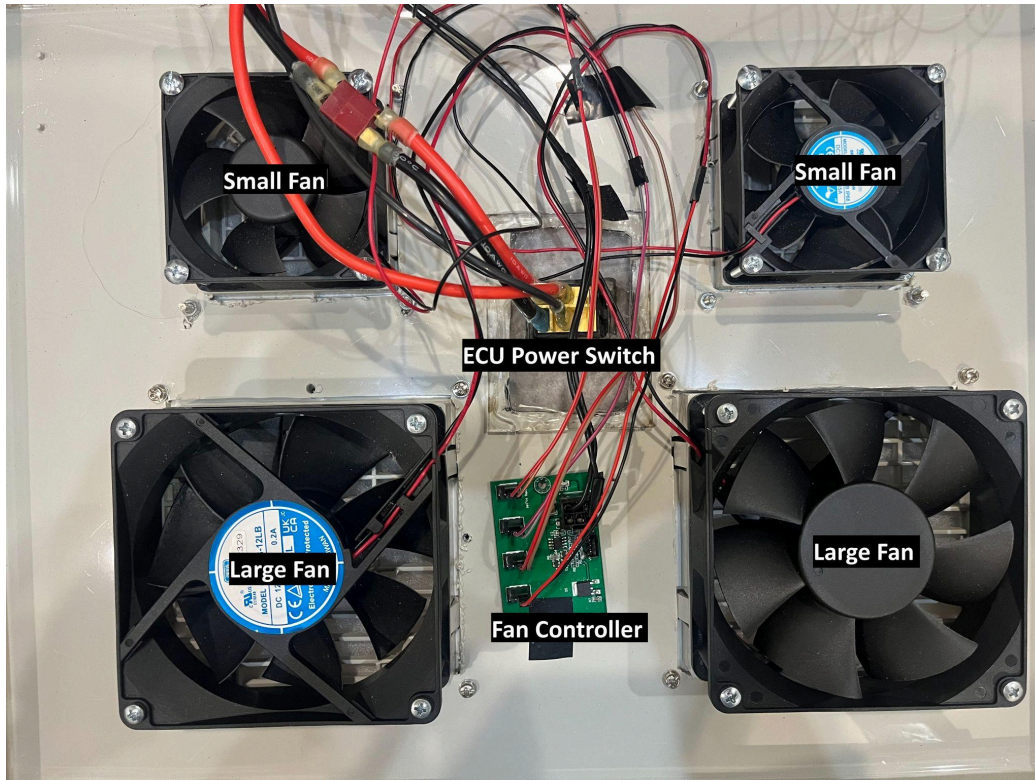
Fig. 17: ECU (Lid)
