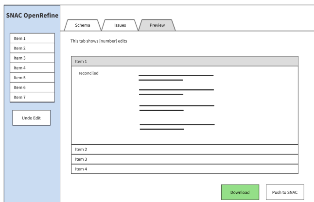
Figure 3.1.1 - Schema Wireframe
